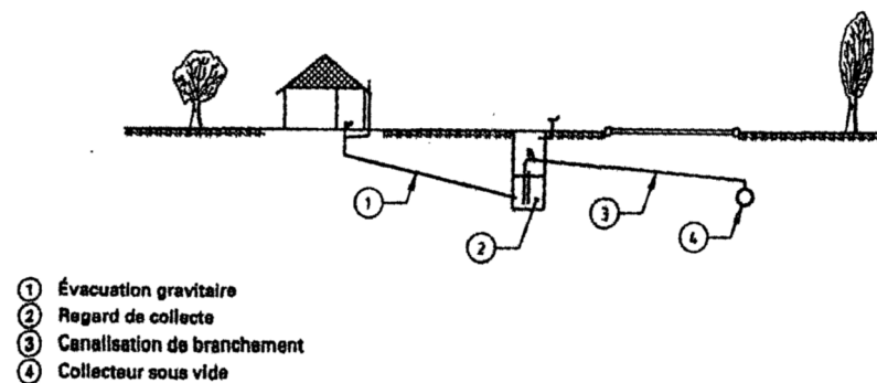
Figure 2 : Branchement d'habitation
